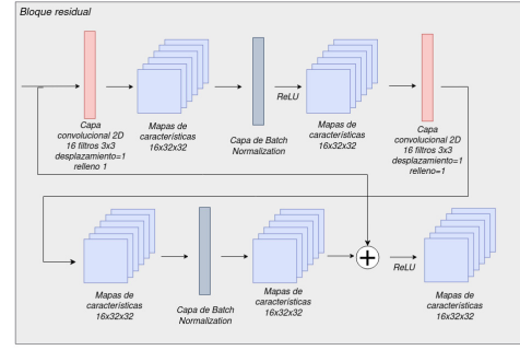
Fig. 4: Ejemplo de bloque residual.
