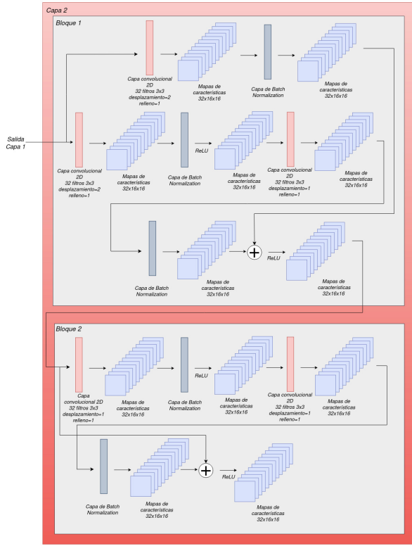
Fig. 6: Capa 2 del codificador ResNet conformada por dos bloques, el primero con reducción de dimensionalidad y el segundo sin esta.
