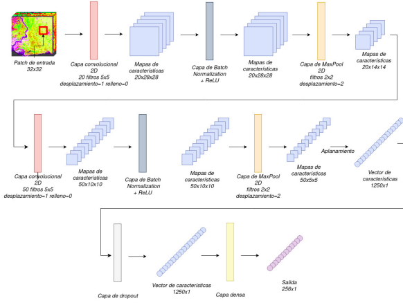
Fig. 3: Diagrama de la estructura del codificador básico.
