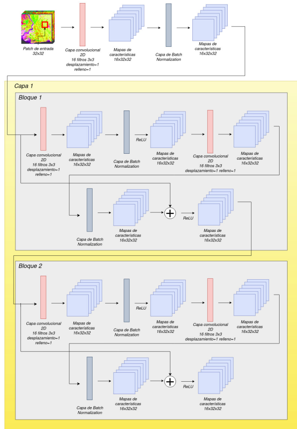
Fig. 5: Capa 1 del codificador ResNet conformada por dos bloques sin reducción de dimensionalidad.
