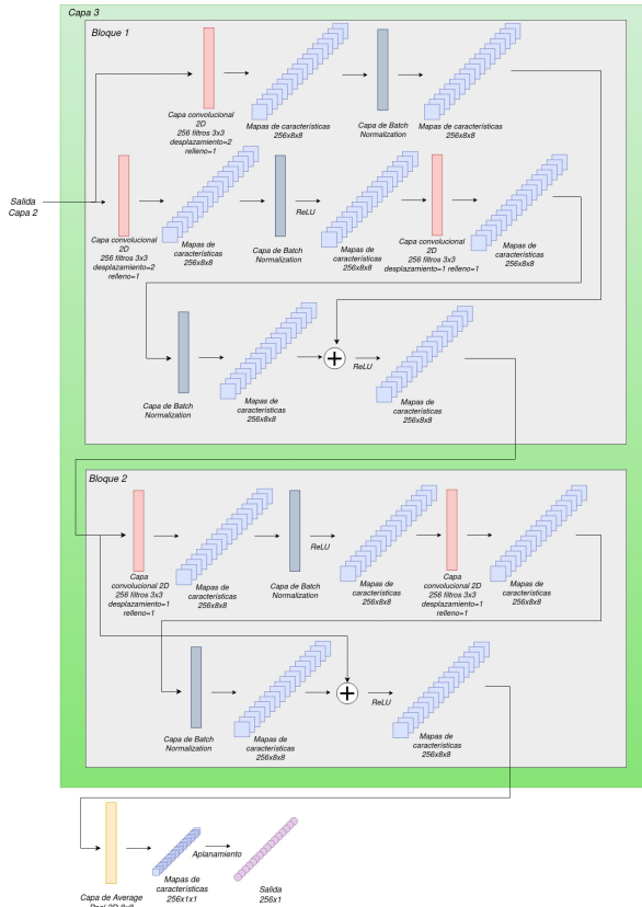
Fig. 7: Capa 3 del codificador ResNet conformada por dos bloques, el primero con reducción de dimensionalidad y el segundo sin esta.
