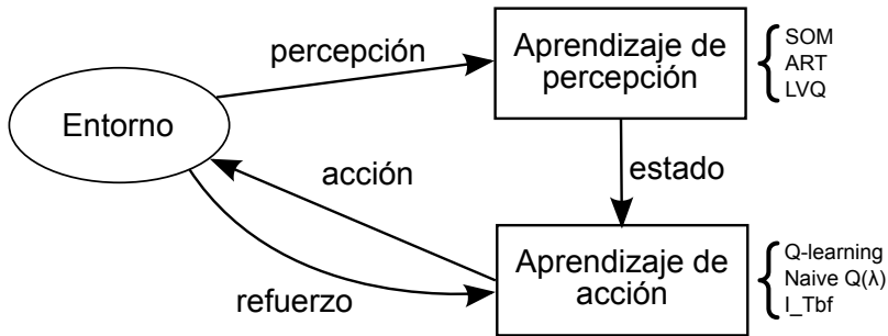
Figura 4.3: Esquema general de nuestra propuesta para el aprendizaje simultáneo de percepción y acción.
