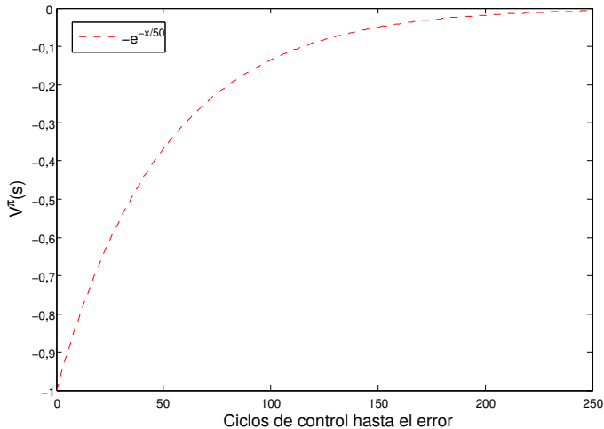
Figura 3.1: Evolución de la función de valor respecto al tiempo estimado de fallo. Los valores del eje x representan Tbf/T , donde Tbf es el tiempo antes del fallo (en segundos) y T es el período de control del robot (en segundos).
